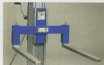
フラットフォーク: アルミニウム製の頑強な作りで、標準的なパレット用です。フォークリフトの代用として経済的なフォークです。SLA-5、10、15モデルで使用可能。オプション
