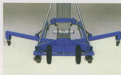
固定スタビライザー: 特許を取得したこのロックシステムにより、重い荷物を側面から支えます。SLA-20、25のユニットに標準装備されています。
