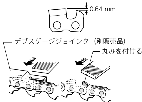
デプスゲージセッティング
