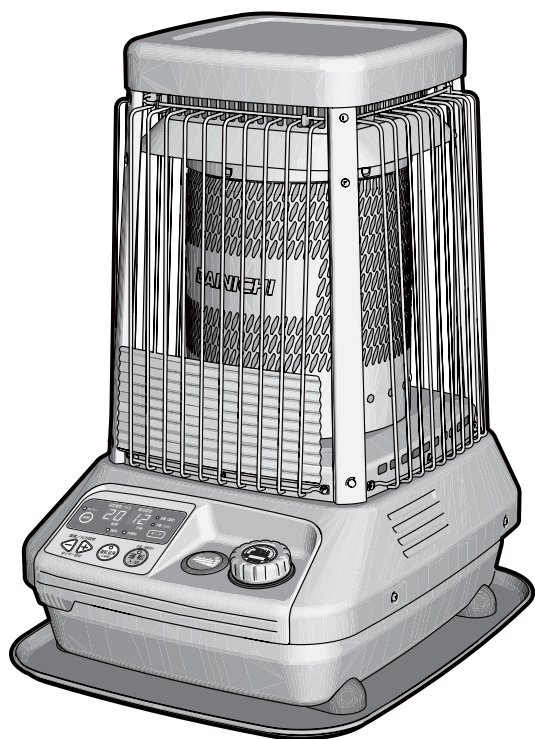
[強制通気形開放式石油ストーブ]
