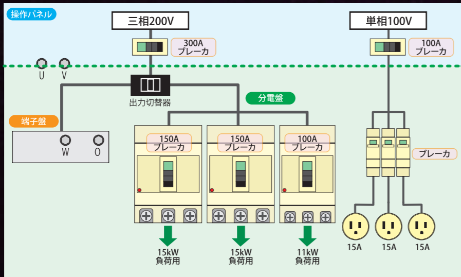
□結線図 SDG100S
